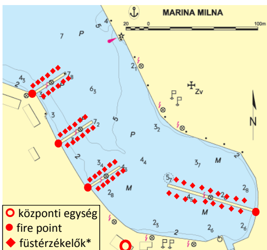
Példamegoldás a 183 férőhelyes ACI Marina Milna-ban (Hotvátó.), *a füstérzékelők kiosztása csak jelképes
